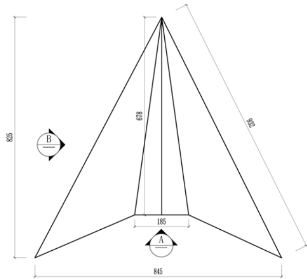
平面图 S=1:8
