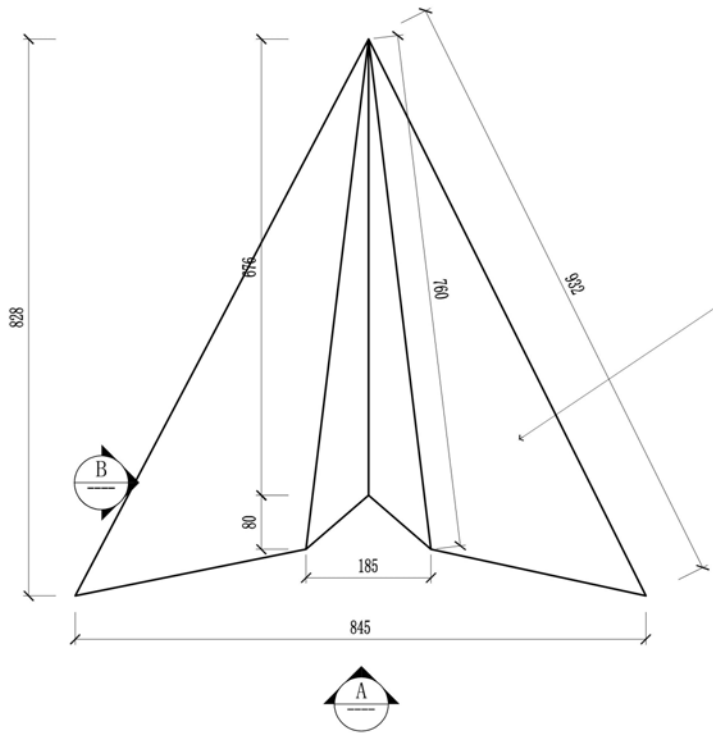
纸飞机平面图 S=1:8
