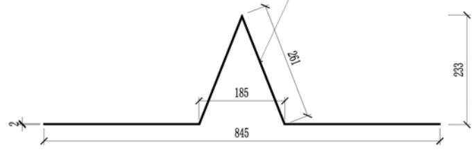
纸飞机A立面图 S=1:8
